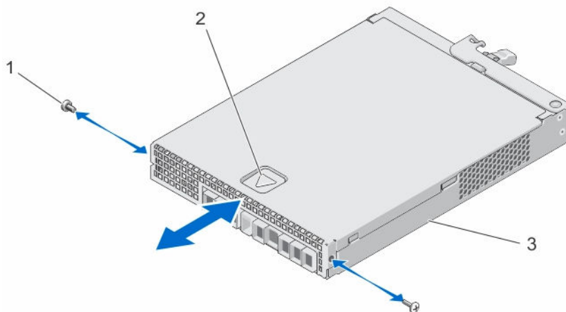
图 21: 打开和关闭 RAID 控制器模块
