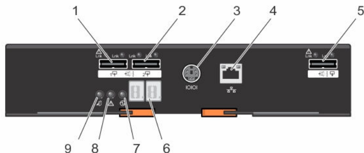
图 9: MD3060e 扩展 模块功能部件和指示灯
