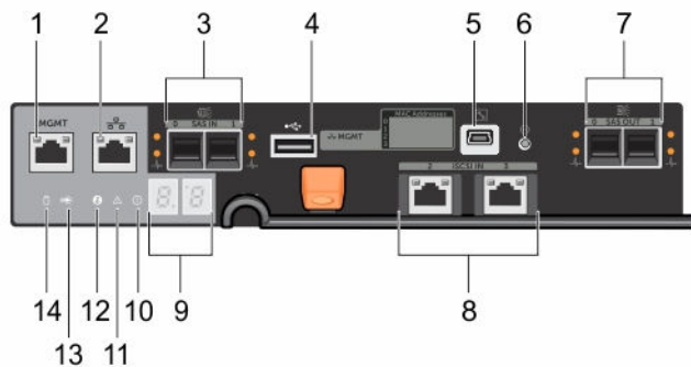
图 8: MD3860i iSCSI RAID 控制器模块功能部件和指示灯
