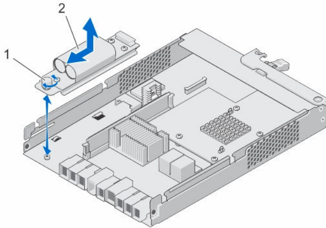
Figure 22. 卸下和 安装 RAID 控制器模块备用电池装置
