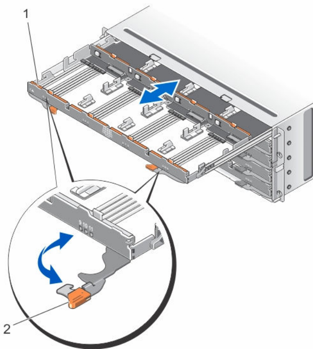
图 12: 打开与合上物理磁盘盘位
