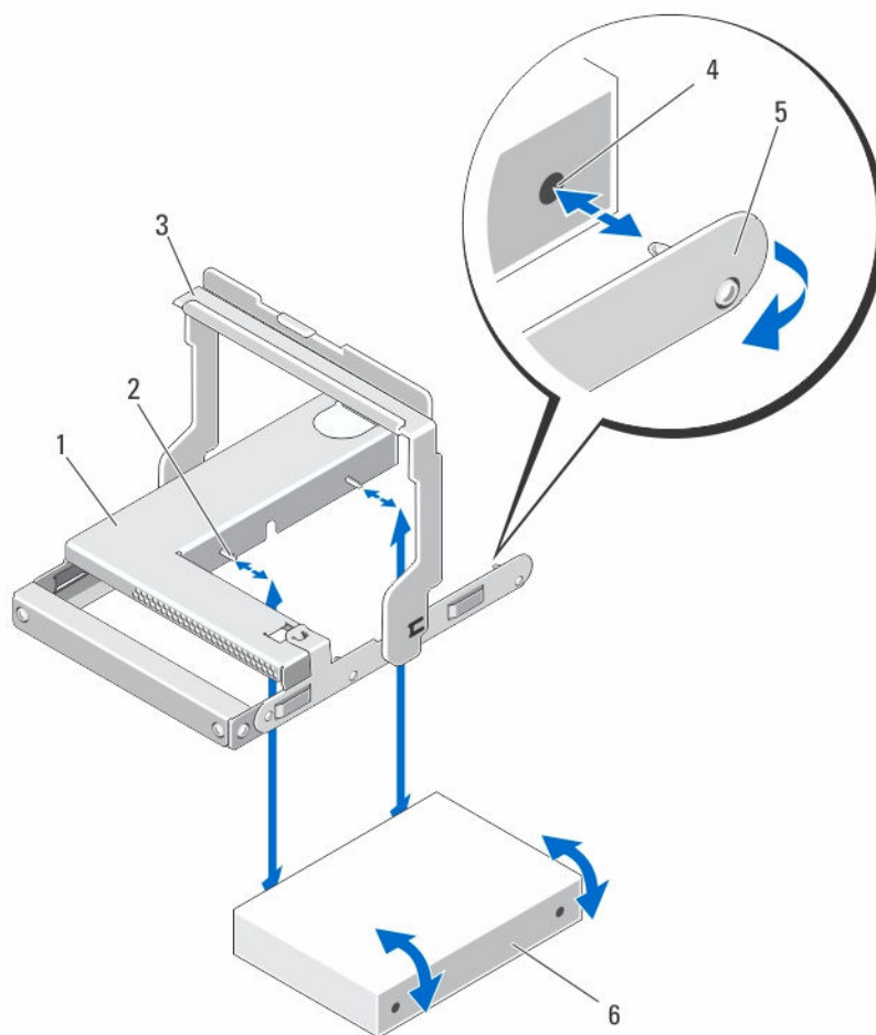
图 15: 在 2.5 英寸物理磁盘托盘中卸下和安装 2.5 英寸物理磁盘
