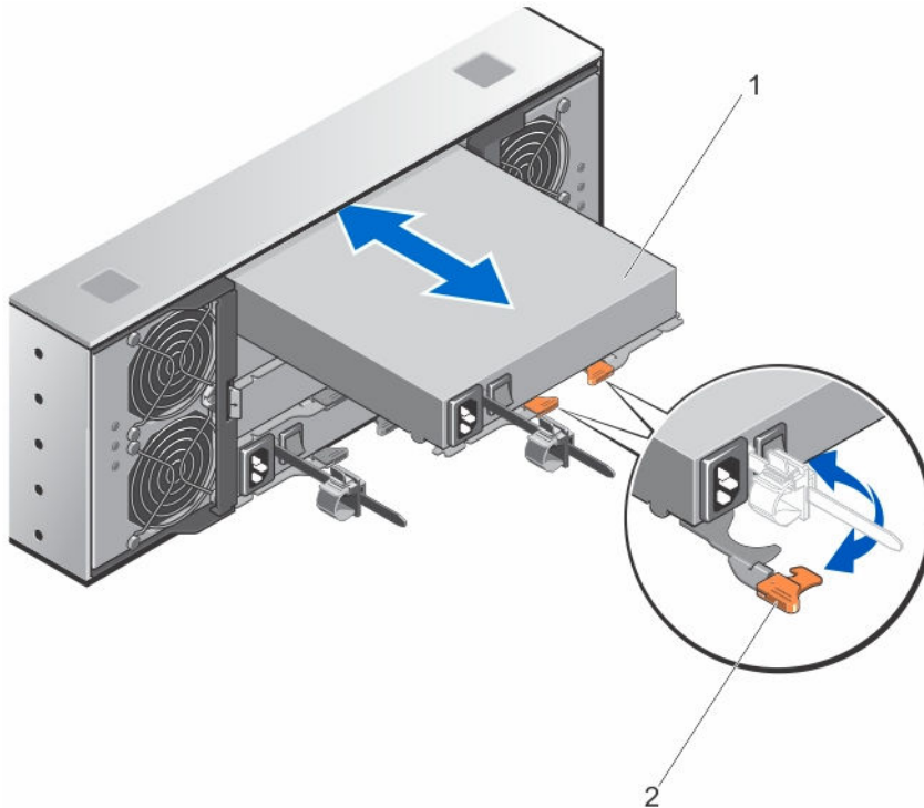
图 23: 卸下和安装电源设备模块
