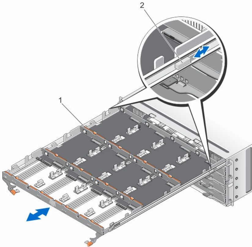
图 13: 卸下和安装物理磁盘盘位
